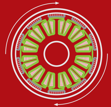
Moteur à rotor extérieur
